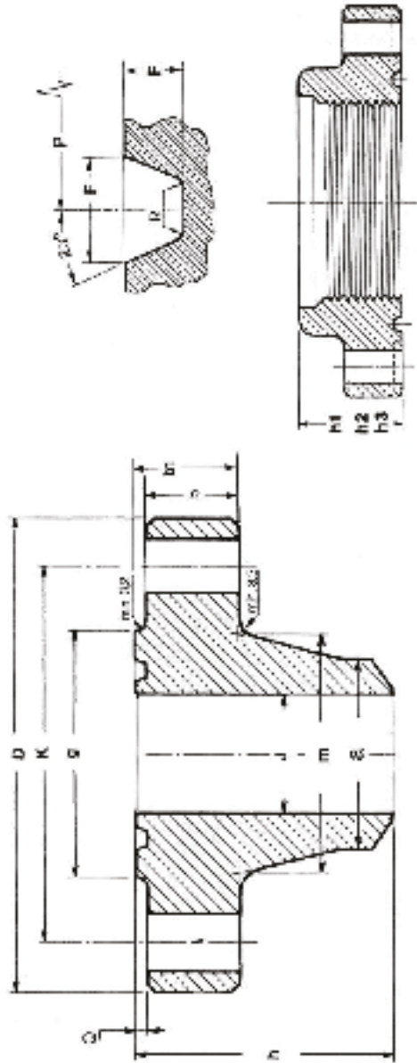
A saldatura di testa - Welding neck
