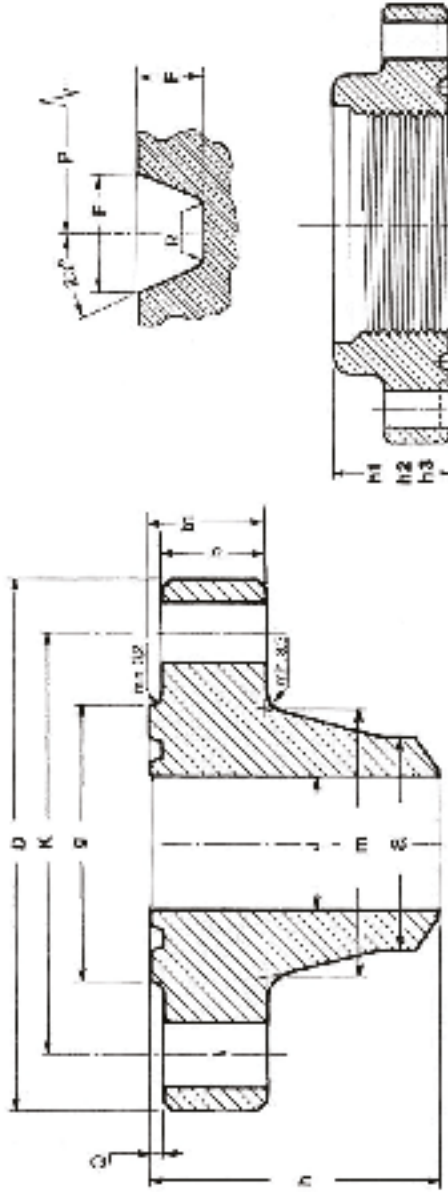
A saldatura di testa - Welding neck
